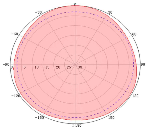
1800MHz Horizontal
