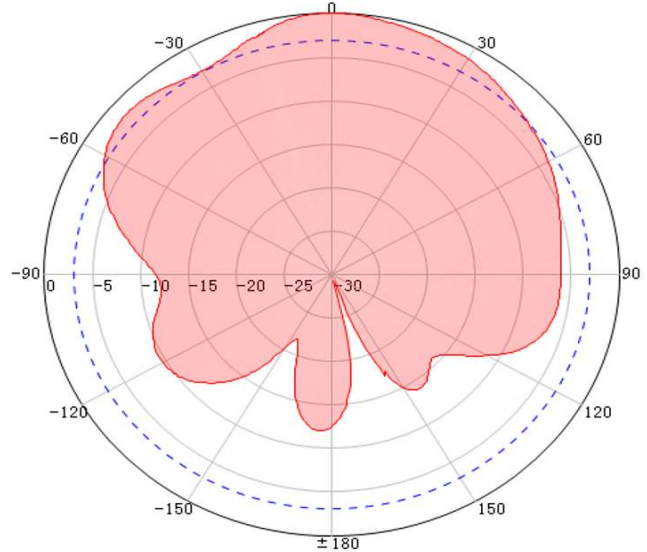
2600MHz Vertical
