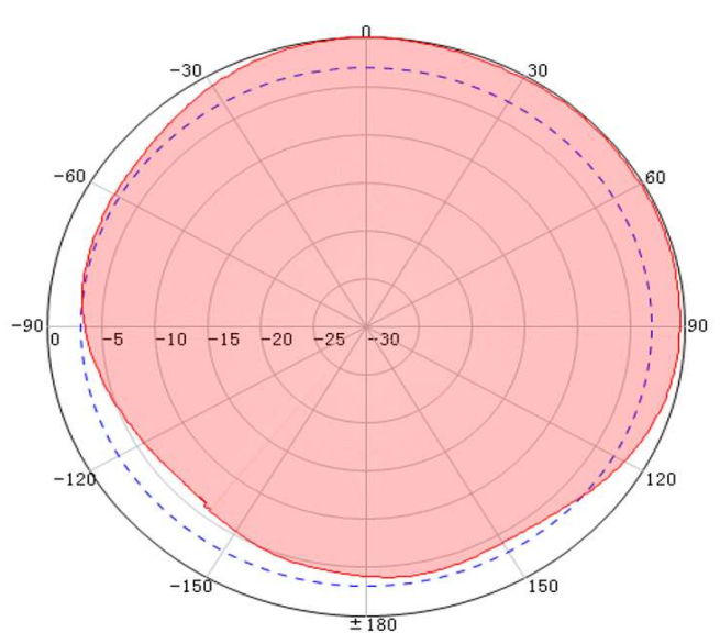
2600MHz Horizontal
