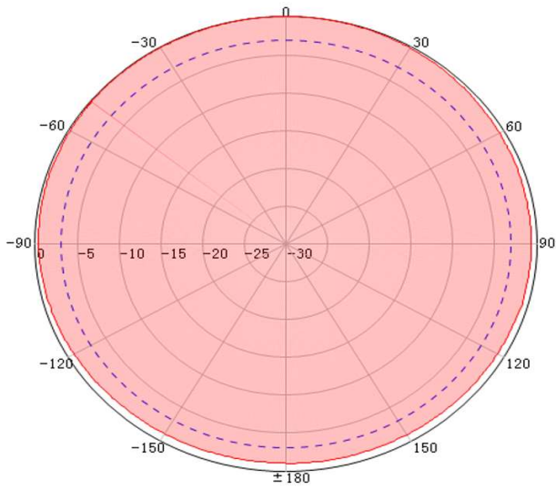
960MHz Horizontal
