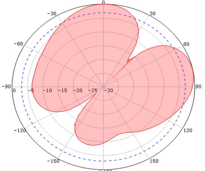
2600MHz Vertical
