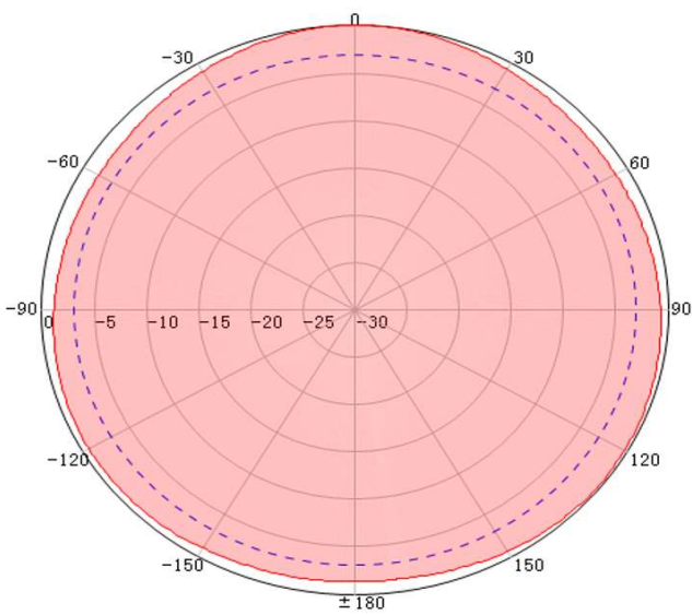
2100MHz Horizontal
