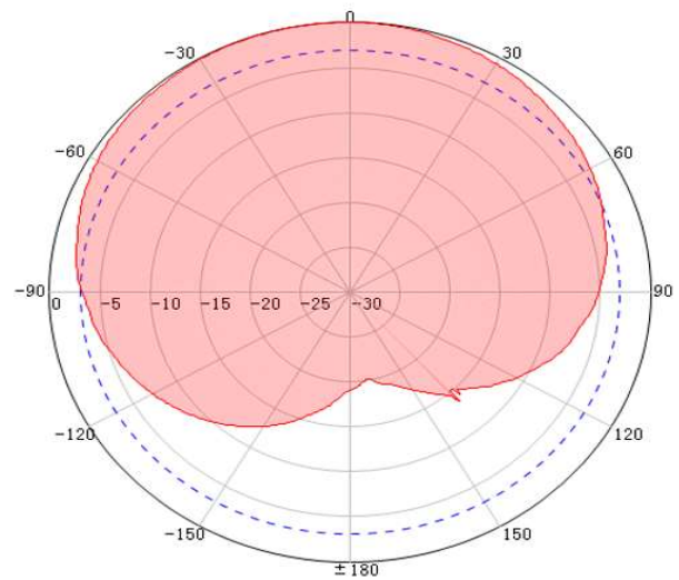
700MHz H Plane
